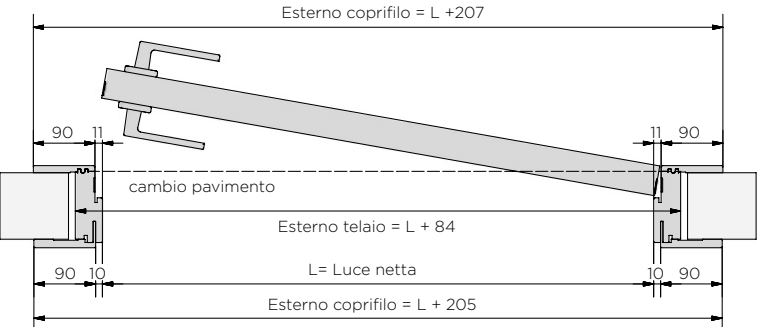
sezione orizzontale
