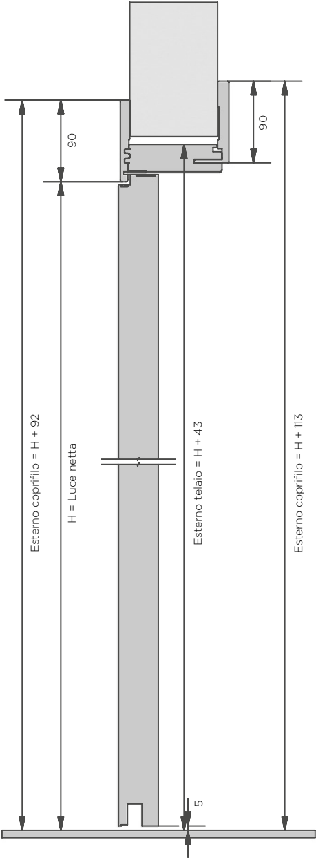
sezione verticale
