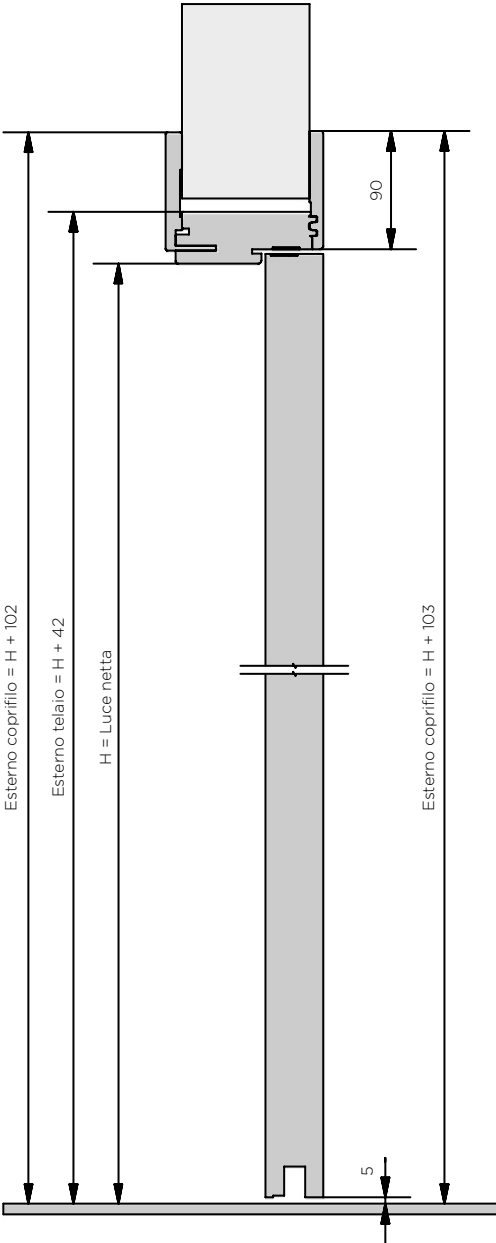
sezione verticale
